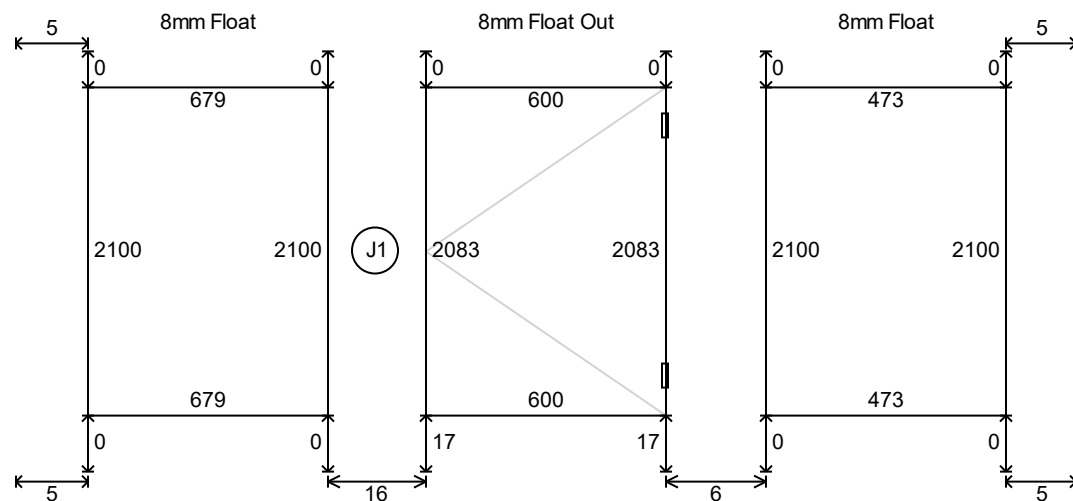
Wymiary Zewnętrzne
