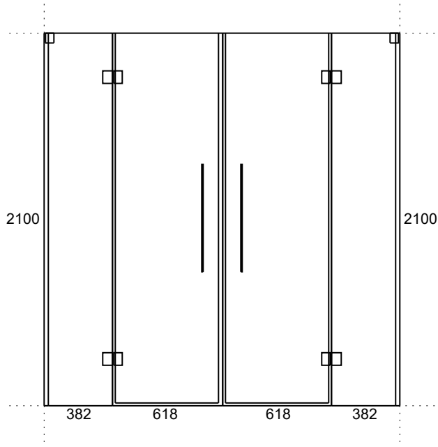
Wymiary Zewnętrzne
