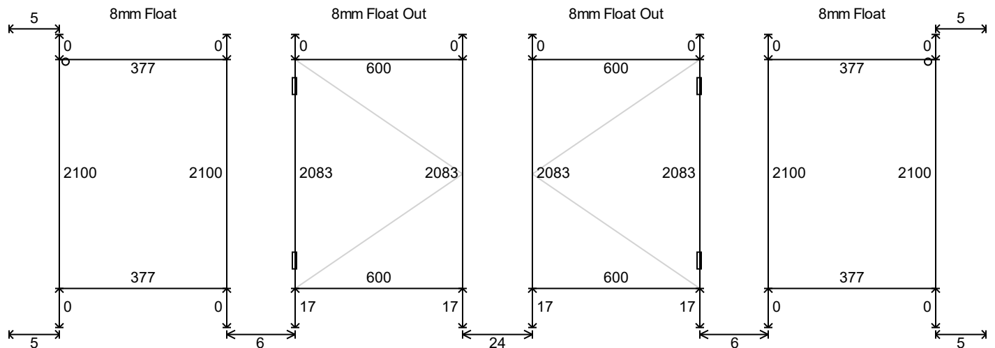
Wymiary Zewnętrzne
