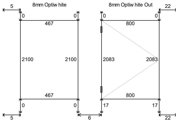
Wymiary Zewnętrzne
