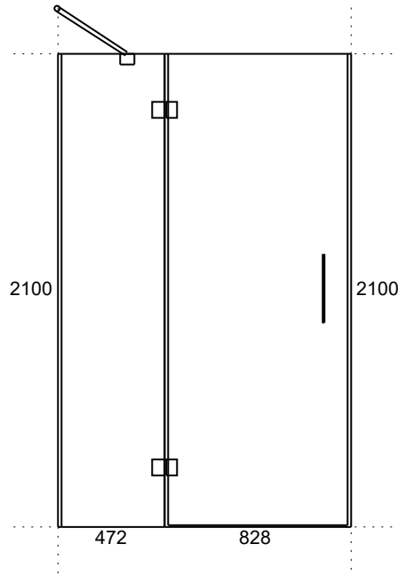
Wymiary Zewnętrzne
