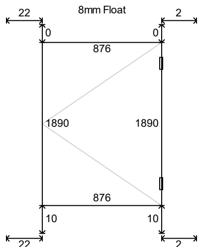
Wymiary Zewnętrzne
