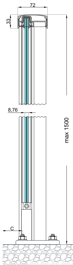
MONTAŻ Z PORĘCZĄ
