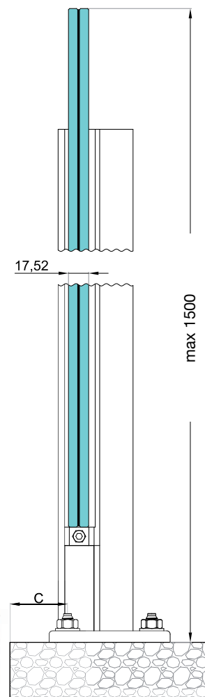
MONTAŻ BEZ PORĘCZY Z KRÓTSZYM SŁUPKIEM
