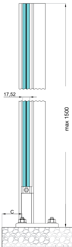
MONTAŻ BEZ PORĘCZY
